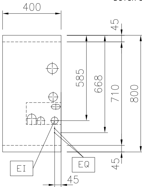
Boven aanzicht
