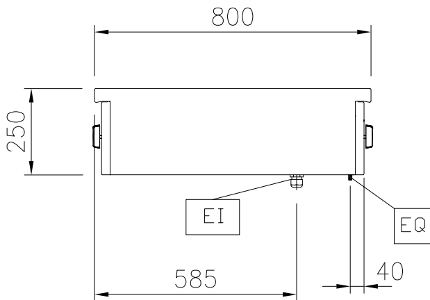
Zij aanzicht
